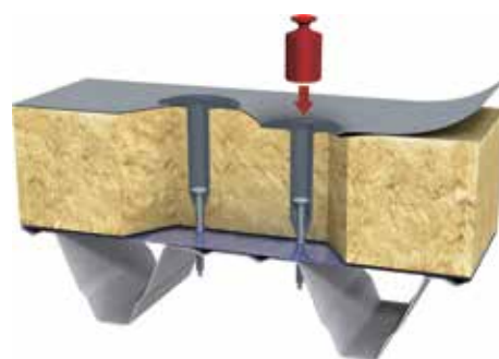
Выдерживает вес человека благодаря телескопической системе
